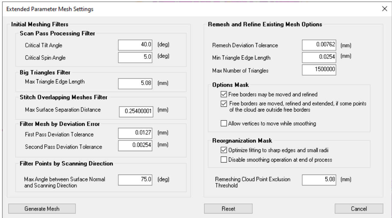
Figure 26-69. Mesh Parameter Controls
